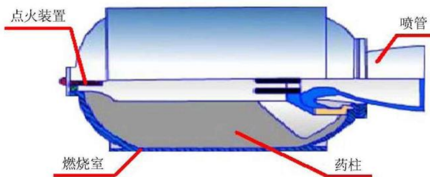
图表11：固体火箭发动机结构示意图
