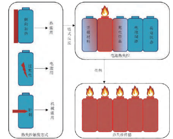
图 31 电池热失控触发方式
