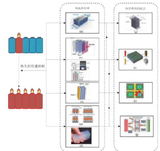
图 32 热管理抑制热失控传播示意图
