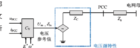
图 29 构网型变流器系统等效图
